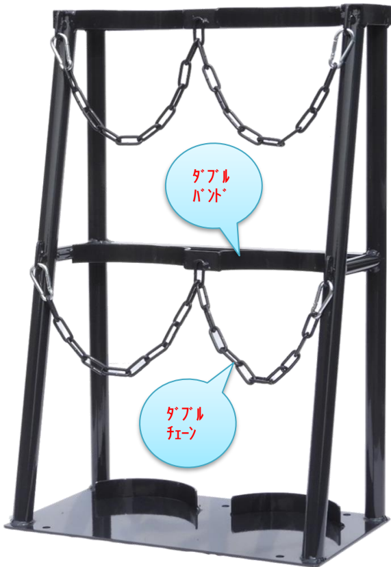
■ ボンベスタンド1500ℓ×2本立上中バンド仕様
